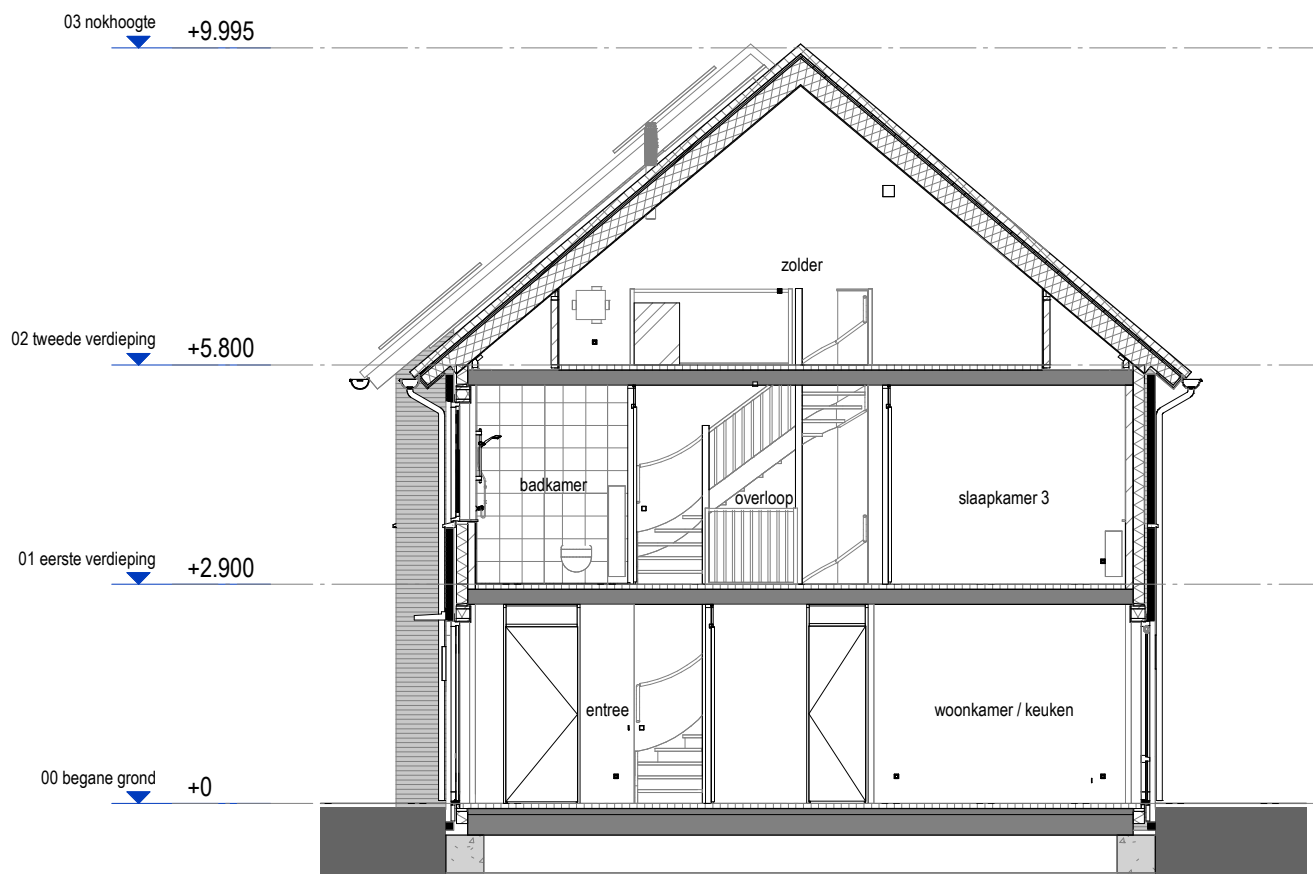
DOORSNEDE 1 : 100
