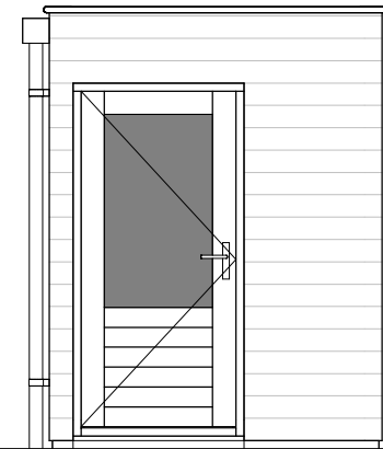
RECHTERGEVEL
